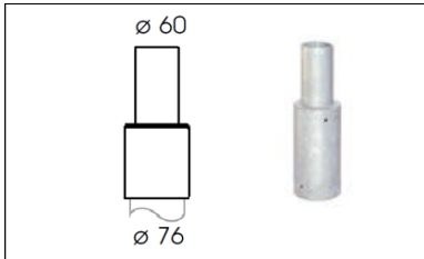
Reduzierungsstück (aufsteckbar) von \varnothing 76 auf \varnothing 60 mm
