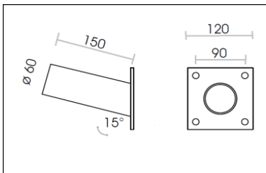
Wandausleger 15° \varnothing 60 mm
