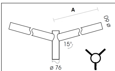
Dreifachausleger 15° für Mastzopf \varnothing 76 mm (aus zylindrischen Rohr)
