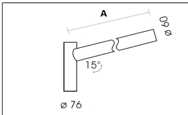
Einfachausleger 15° für Mastzopf \varnothing 76 mm (aus zylindrischen Rohr)
