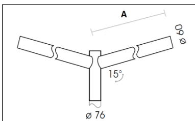
Doppelausleger 15° für Mastzopf \varnothing 76 mm (aus zylindrischen Rohr)
