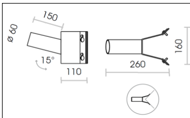
Eckausleger 15° \varnothing 60 mm
